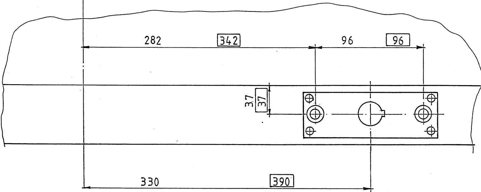
Ansicht "Z"
